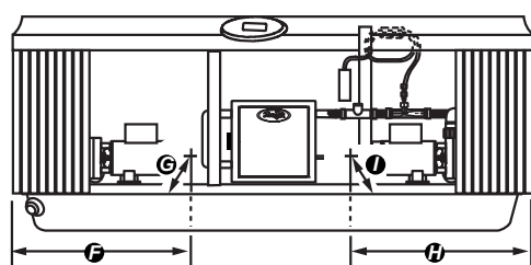
*Bottom Conduit Port Access Dimensions - Optional
